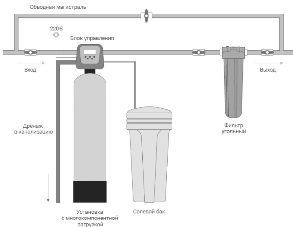
Схема комплекта водоочистки "Стандарт"
