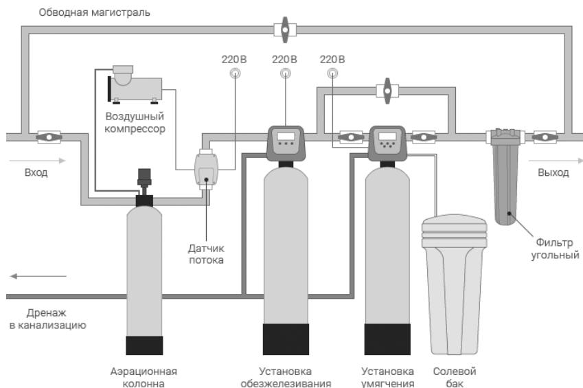
Схема комплекта водоочистки "Оптимум"
