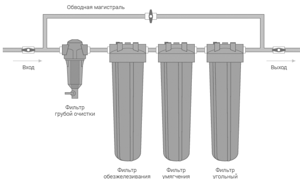
Схема комплекта водоочистки "Эконом"
